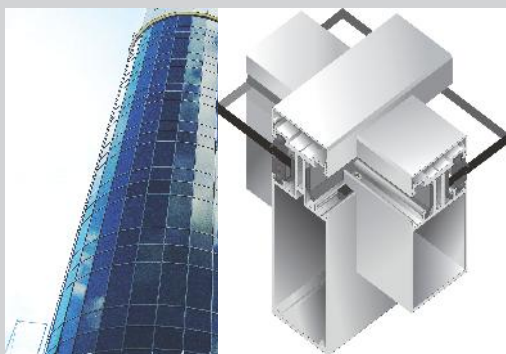
Система КП50К
